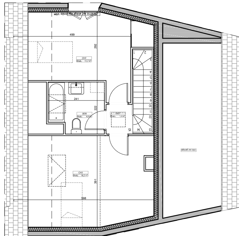
plan du R+1 - 1/100°
