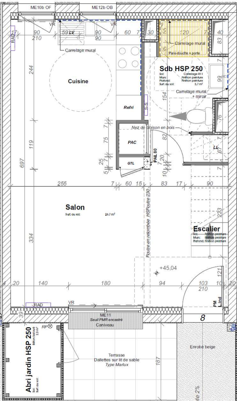
REZ-DE-CHAUSSEE
