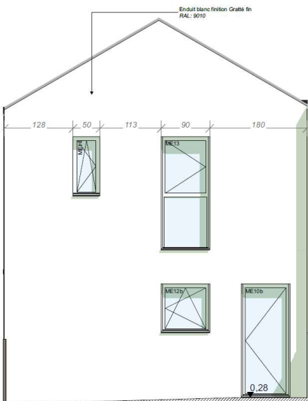
FAÇADE NORD-EST
